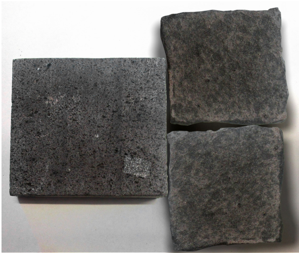
Innenstadt Mobilitätsstreifen Basaltlava - Oberfläche diamantgeschliffen Neupflaster Basalt
