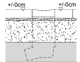
EW 12 Offene Rinne, Straßeneinlauf
