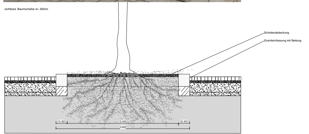
Schnitt Baumscheibe (Bestandsbaum)
