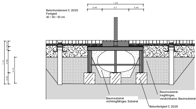
Schnitt Baumscheibe Unterflurbaumrost (Neupflanzung)
